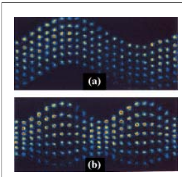
圖七：7個陷獲離子的集體運動：(a)質心模；(b)呼吸模。(本圖取自 Innsburck 大學物理系)
