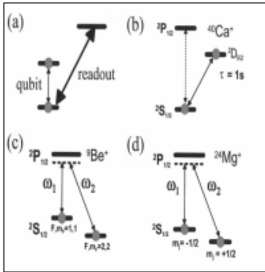
圖四：適用於量子計算的陷獲離子之能階結構圖。 (本圖取自參考資料[2])
