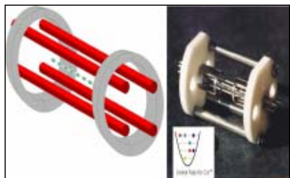
圖六：Innsburck 大學所設計使用的線性離子阱外觀及構造。(本圖取自 Innsburck 大學物理系)
